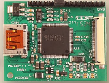
MCIB-11
